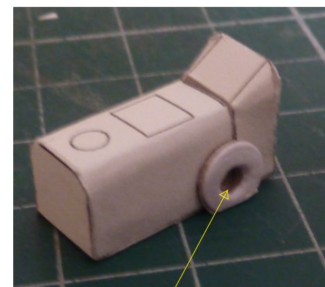
Mettez ici l'essieu B3
